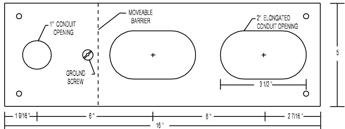
FA6 - FM6 BASE
