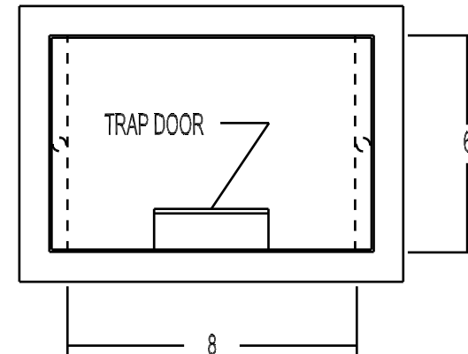
LID DETAIL
