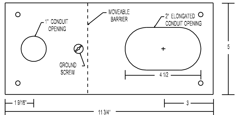
FA5 - FM5 BASE
