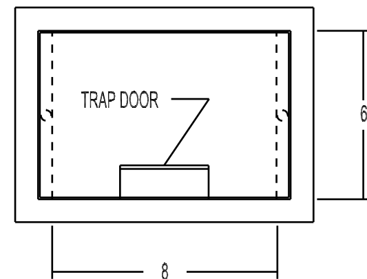
LID DETAIL
