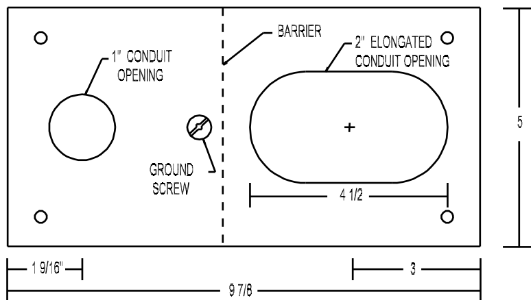
FA4 - FM4 BASE
