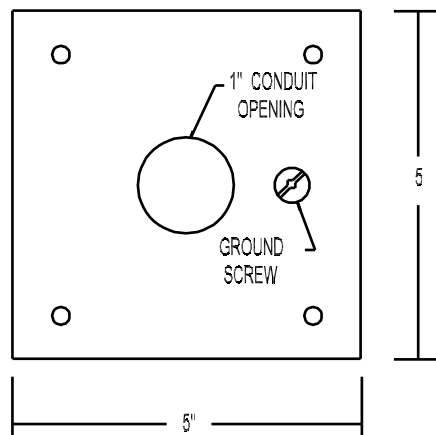
FA2 - FM2 BASE
