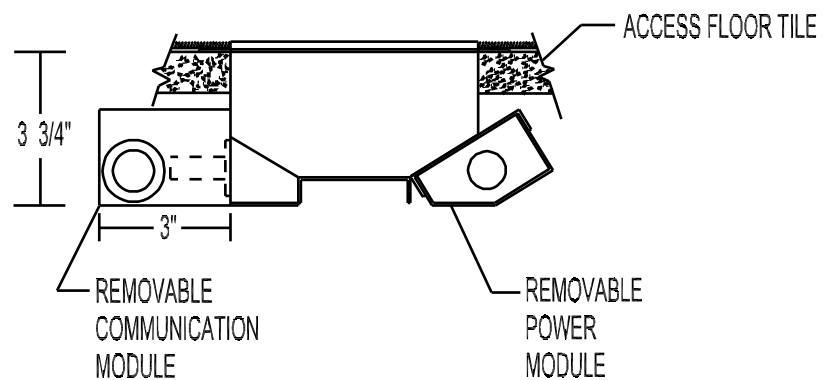
LID DETAIL
